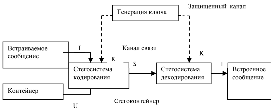
Рисунок 1- Структура стеганографической системы
