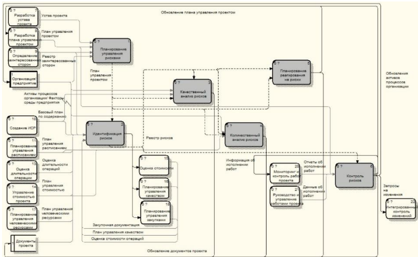
Рисунок 3 - Диаграмма DFD
