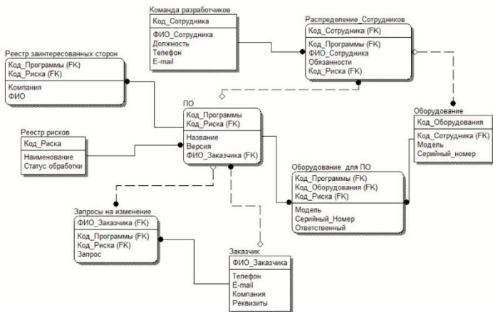
Рисунок 5 - Диаграмма IDEF1X
