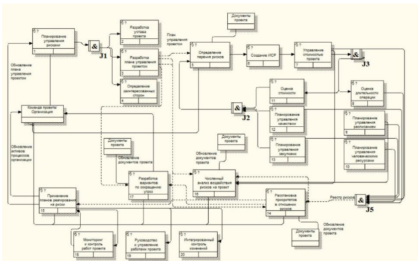
Рисунок 4 - Диаграмма IDEF3
